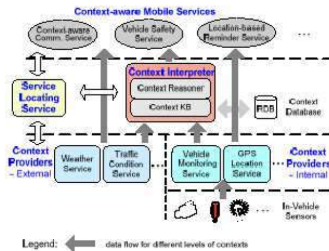
Figura 3.3: Arquitetura do SOCAM
