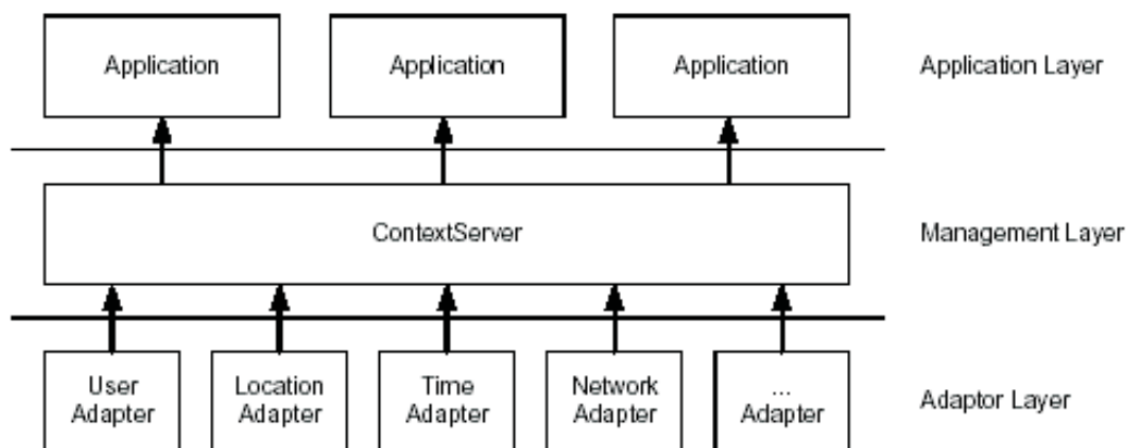
Figura 3.8: Arquitetura do Hydrogen
