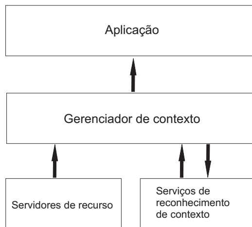
Figura 3.2: Arquitetura do Context Managing Framework
