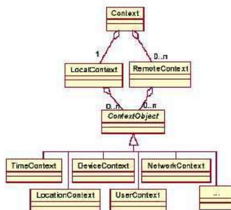
Figura 3.7: Gerenciamento de Contextos Local e Remoto do Hydrogen
