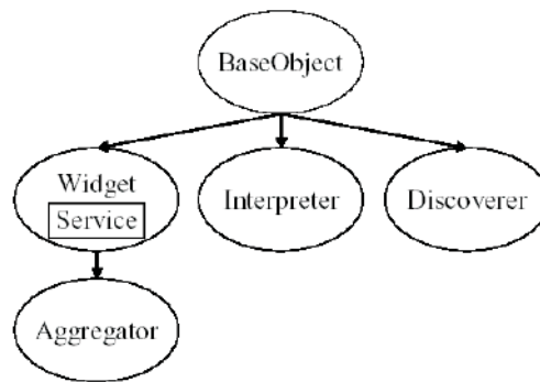
Figura 3.6: Abstrações do Context Toolkit
