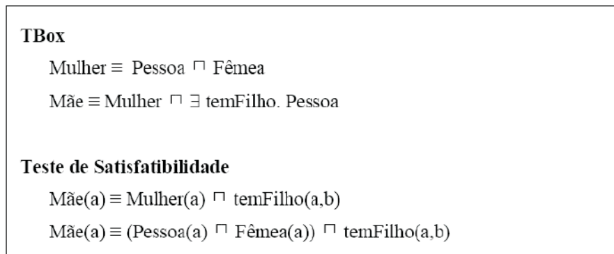
Figura 4.5: Teste de Satisfatibilidade
