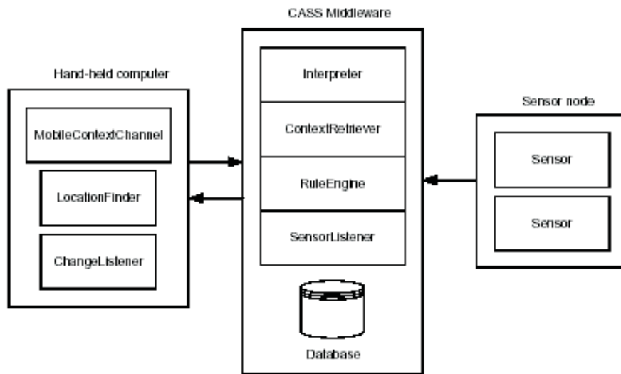
Figura 3.4: Arquitetura do CASS
