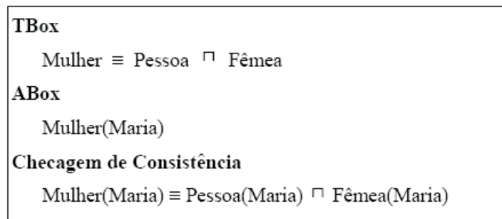
Figura 4.9: Checagem de Consistência
