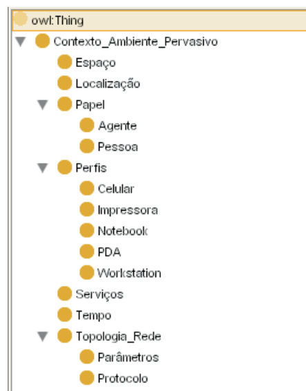
Figura 5.5: Ontologia do contexto do ambiente pervasivo
