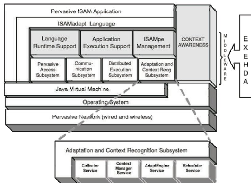
Figura 2.6: Subsistema de Reconhecimento de Contexto e Adaptação do EXEHDA
