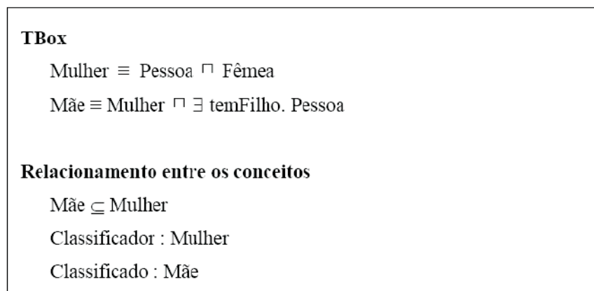
Figura 4.6: Teste de Subclassificação
