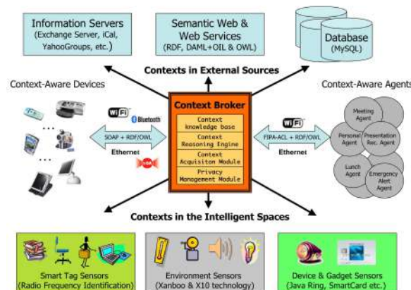
Figura 3.5: Arquitetura do CoBrA
