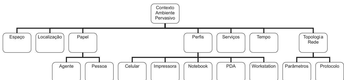
Figura 5.3: Árvore de classificação de conceitos da ontologia do contexto do ambiente pervasivo
