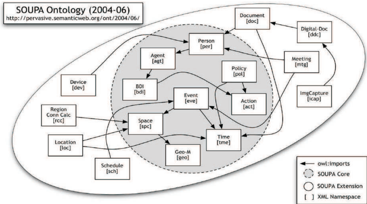
Figura 5.1: Ontologia SOUPA
