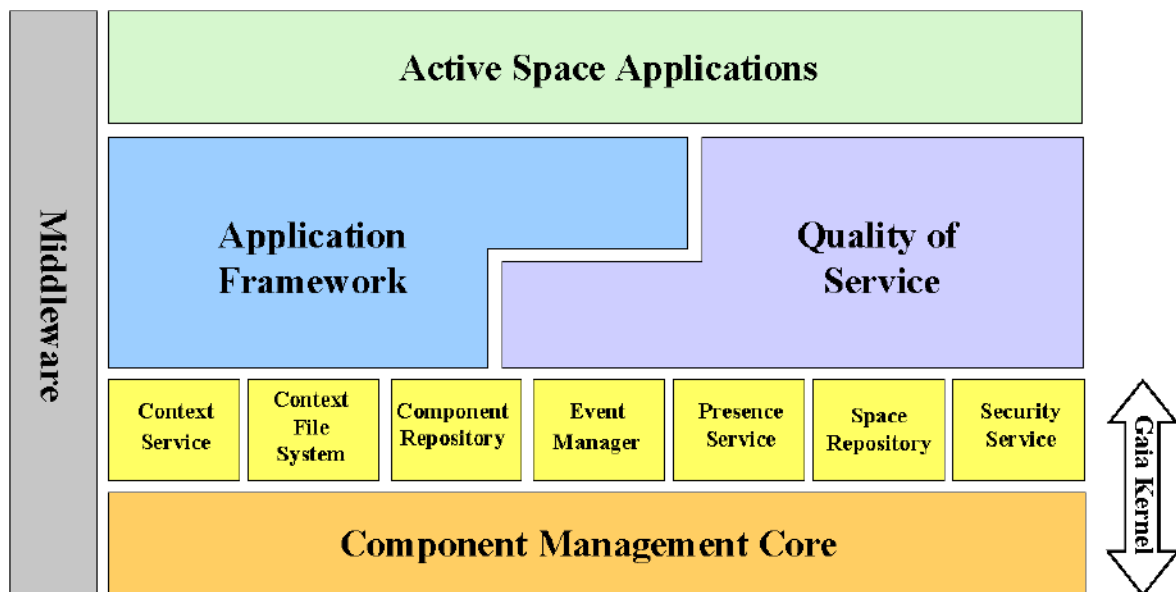
Figura 2.2: Arquitetura do Gaia
