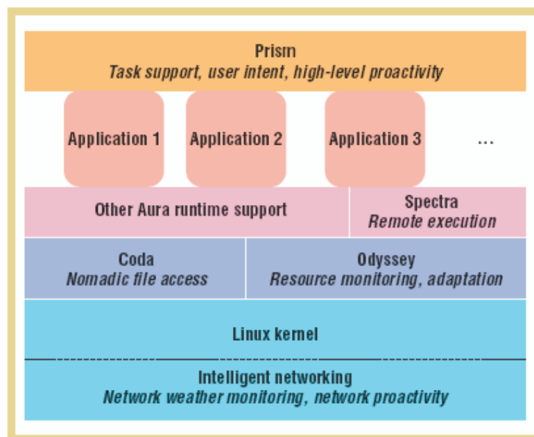
Figura 2.3: Arquitetura do Projeto Aura
