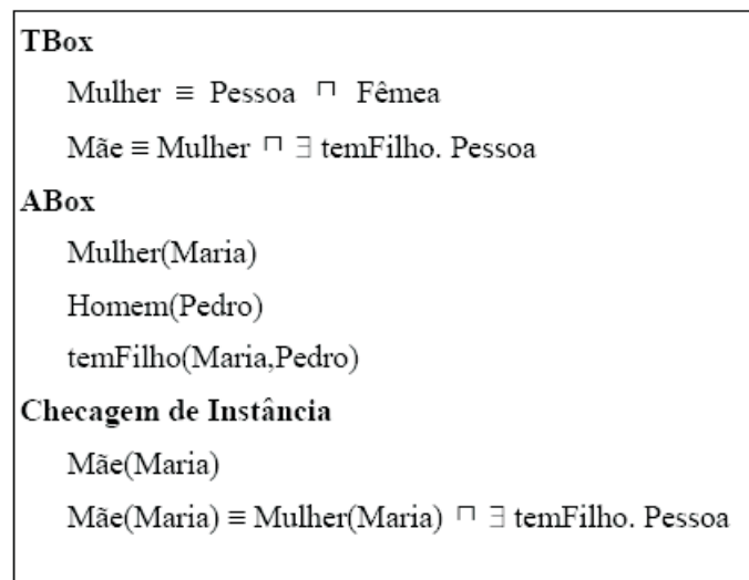
Figura 4.10: Checagem de Instância
