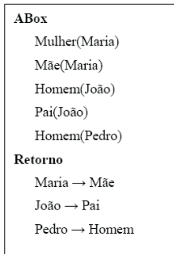
Figura 4.11: Serviço de Retorno do RACER
