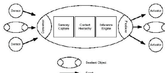
Figura 3.9: Modelo de Objeto do CORTEX
